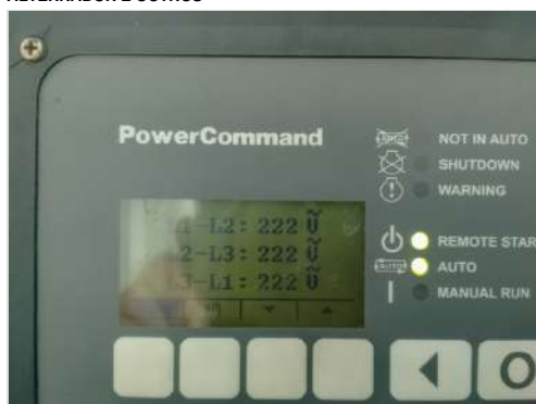
FOTOS DA TENSÃO DA BATERIA, FREQUÊNCIA, TENSÃO GERADA NO ALTERNADOR E OUTROS
