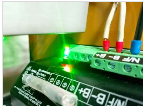
FOTOS DO QUADRO DE COMANDO INTERNO, GRUPO GERADOR (MOTOR E ALTERNADOR)
